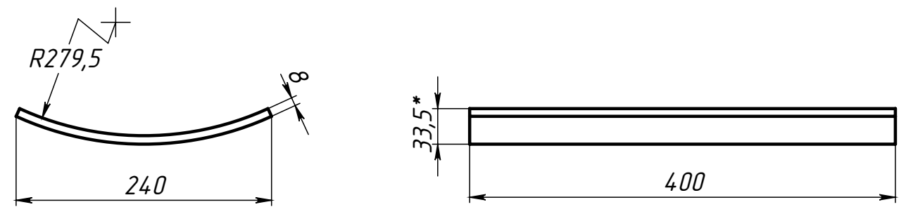
Поз.3 (Ложемент)
